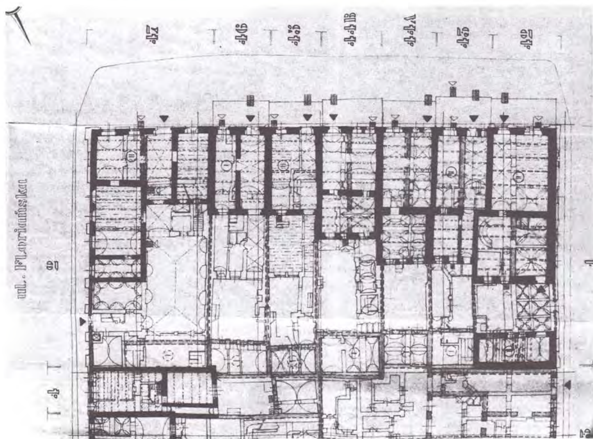
Ryc. 3. Rekonstrukcja bloku zabudowy mieszkalnej między Rynkiem Głównym i ul. Floriańska, św. Jana i św. Tomasza, część południowa, parter. Stan w 2. poł. XIV w. Opr. M. Łukacz w 1982 r.
