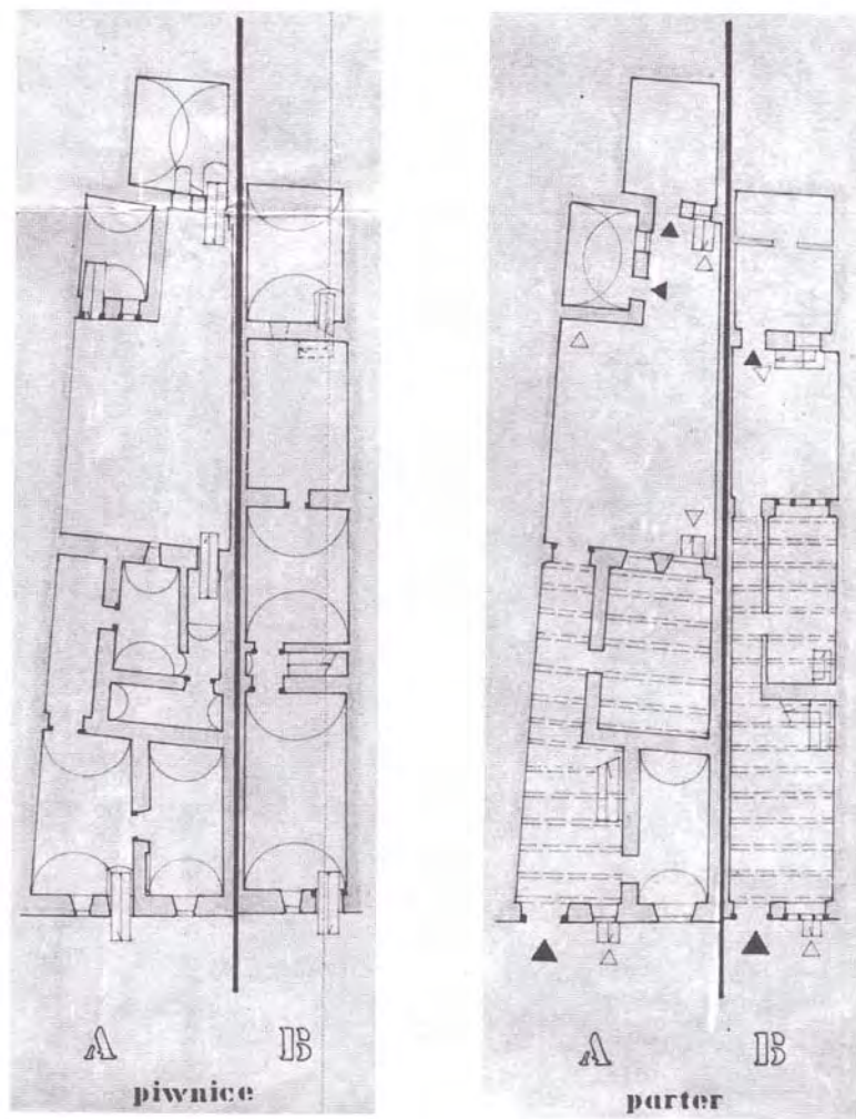
Ryc. 5. Rekonstrukcja rzutu piwnic i parteru kamienic tworzących od 1830 r. obecny dom RG 13. Stan w końcu XV w. Opr. A. Karbowski w 1978 r.
