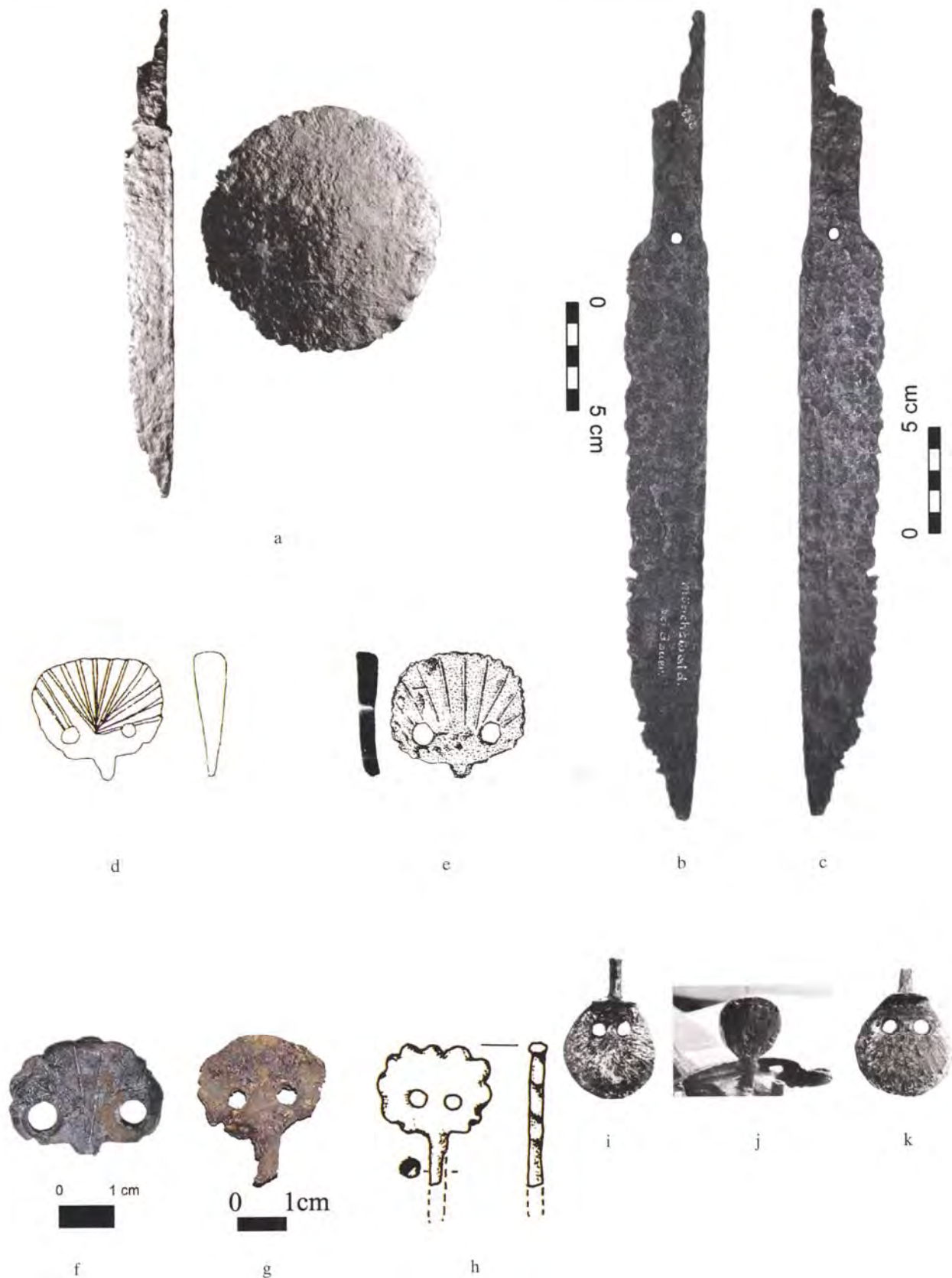
Ryc. 47. a, b, c – kord, 1 poł XV w., Górzec koło Męcinki, pow. jaworski, Muzeum Regionalne w Jaworze, nr inw. 282 A. (a – wg AP WSPŚ, sygn. 716); b-c – fot. L. Marek; d-k – tarczki boczne pugałów i kordów w kształcie muszli św. Jakuba: d – Nowe Miasto Korczyn (za Kajzerem i Rychterem 1997); e – zamek Vartnov, okr. Opava (za Kouřilem i inn. 2001); f-g – zamek Bardo, pow. ząbkowicki, znalezione przy wieży ostatecznej obrony. Fot. L. Marek; h – Jarocin (za Grygielem 1994); i – Republika Czeska, znalezisko luźne; j – przy kordzie z Janosławic, okr. Šumperk, k – zamek Šostýn (i-k – za Michną 1997)
