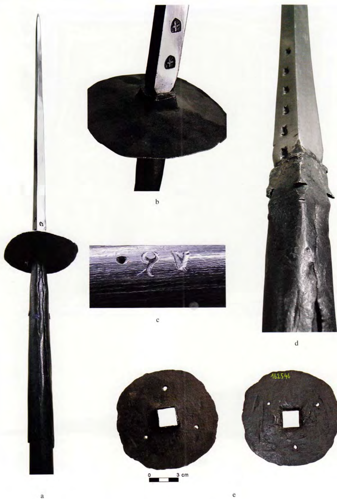
Ryc. 144. Spisy szydlowate z arsenału miasta Wiednia, produkt Hansa Maidburgera z Piesting w Dolnej Austrii, 1497-1500 r. Museum der Stadt Wien: a-c – nr inw. 126.008; d – nacięcia służące do mocowania tarczy (brak widocznego nr. inw.); e – tarcza ochronna, nr inw. 162546, awers i rewers; a-e – fot. L. Marek
