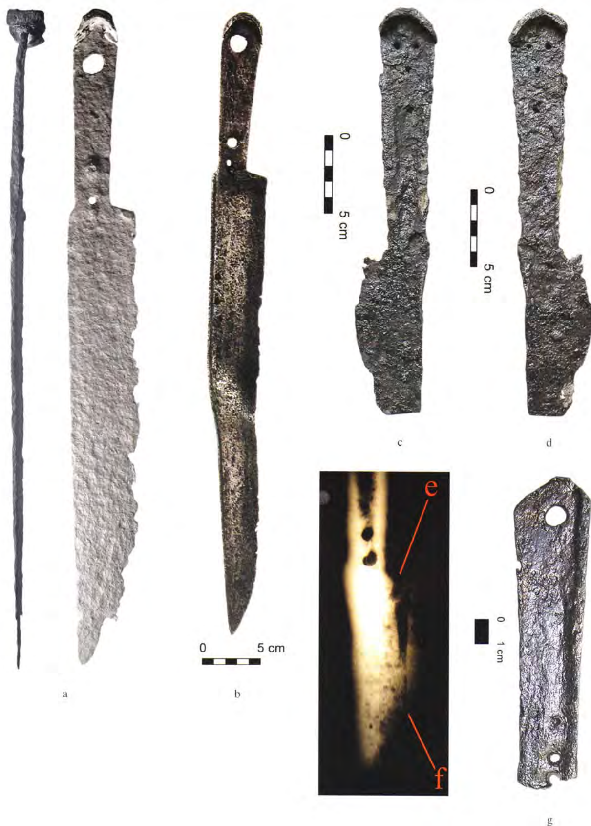
Ryc. 48. Kordy typu II: a – Biskupin pow. legnicki, XV w. (za AF/MAW, nr negatywu 5917), b – Polska Cerekiew pow. kędzierzyński, XV w., Muzeum w Raciborzu, nr inw. MRB97 (fot. T. Gąsior); c-f – zamek Sokolec na Górze Krzyżnej, pow. jeleniogórski XV w., Instytut Archeologii UW; c-d – fot. L. Marek; e – zdjęcie RTG: miejsce dokucia nawęglonej nakładki tworzącej ostrze; g – trzpień kordu o prostopadłe zagiętym grzbiecie, zamek Szczerba koło Gniewoszowa, pow. kłodzki, 1. poł. XV w. Fot. L. Marek
