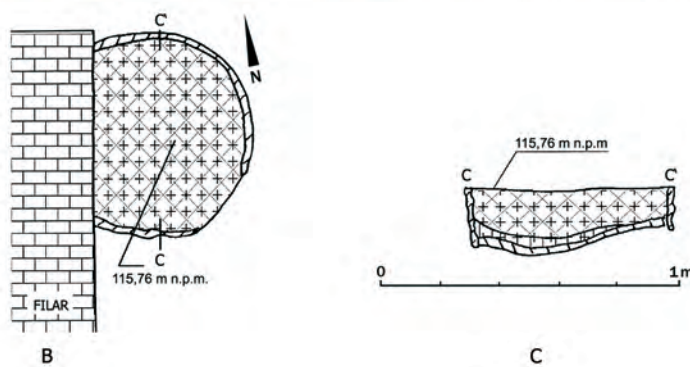
Ryc. 42. Ul. Biskupia 1a, sekt. 2, ob. 4 – kosz z uszczelnionym gliną dnem.
