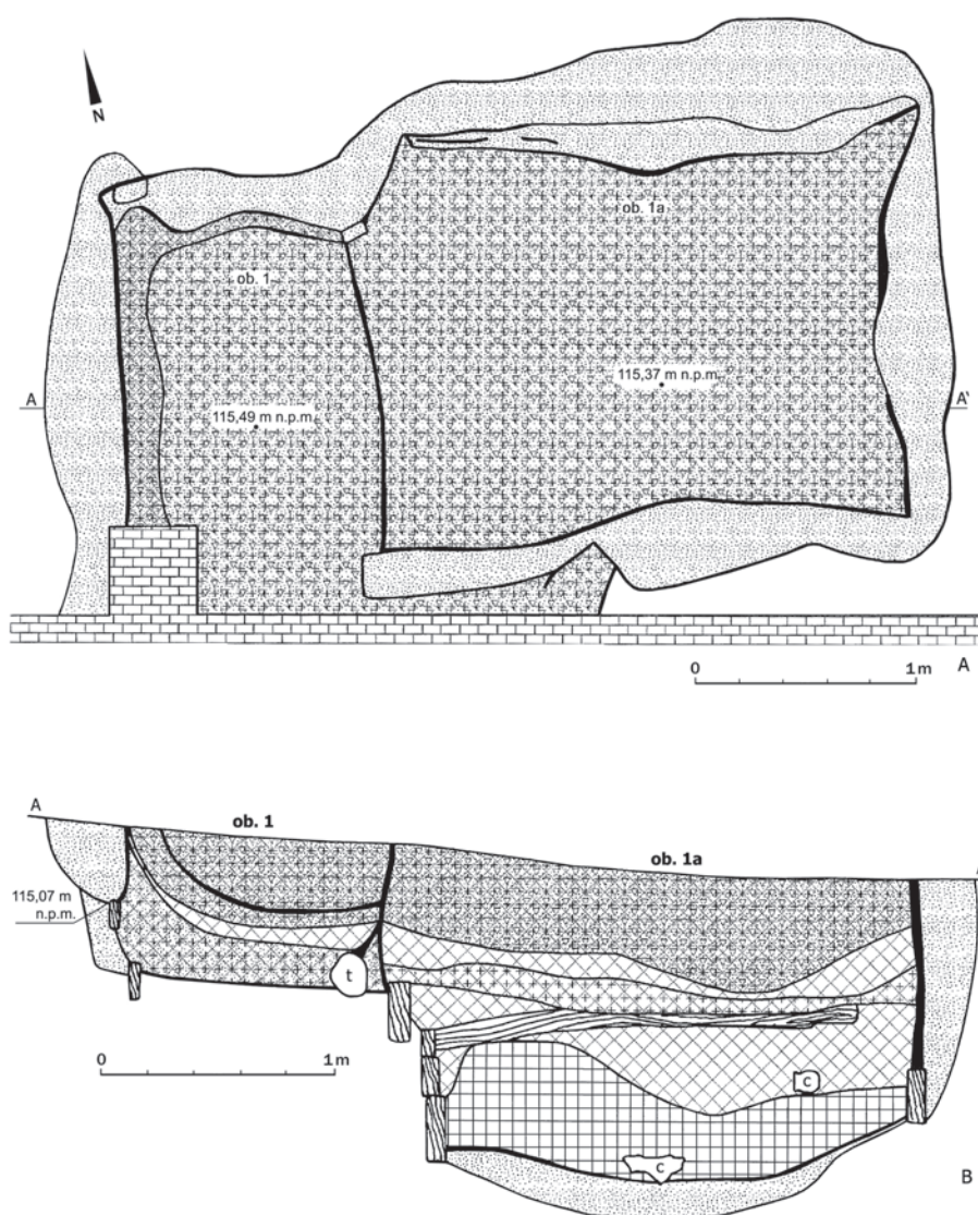
Ryc. 63. Ul. Wierzbowa 3, sektor 2. Kloaka (ob. 1a) wkopana w starszą ziemiankę (ob. 1). Rzut i profil. Wg M. Babija i in. (2001) Abb. 63. Weidenstraße 3, Sektor 2. Kloake (Ob. 1a) in der älteren Erdgrube (Ob. 1). Grundriss und Profil. Nach M. Babij et alii (2001)
