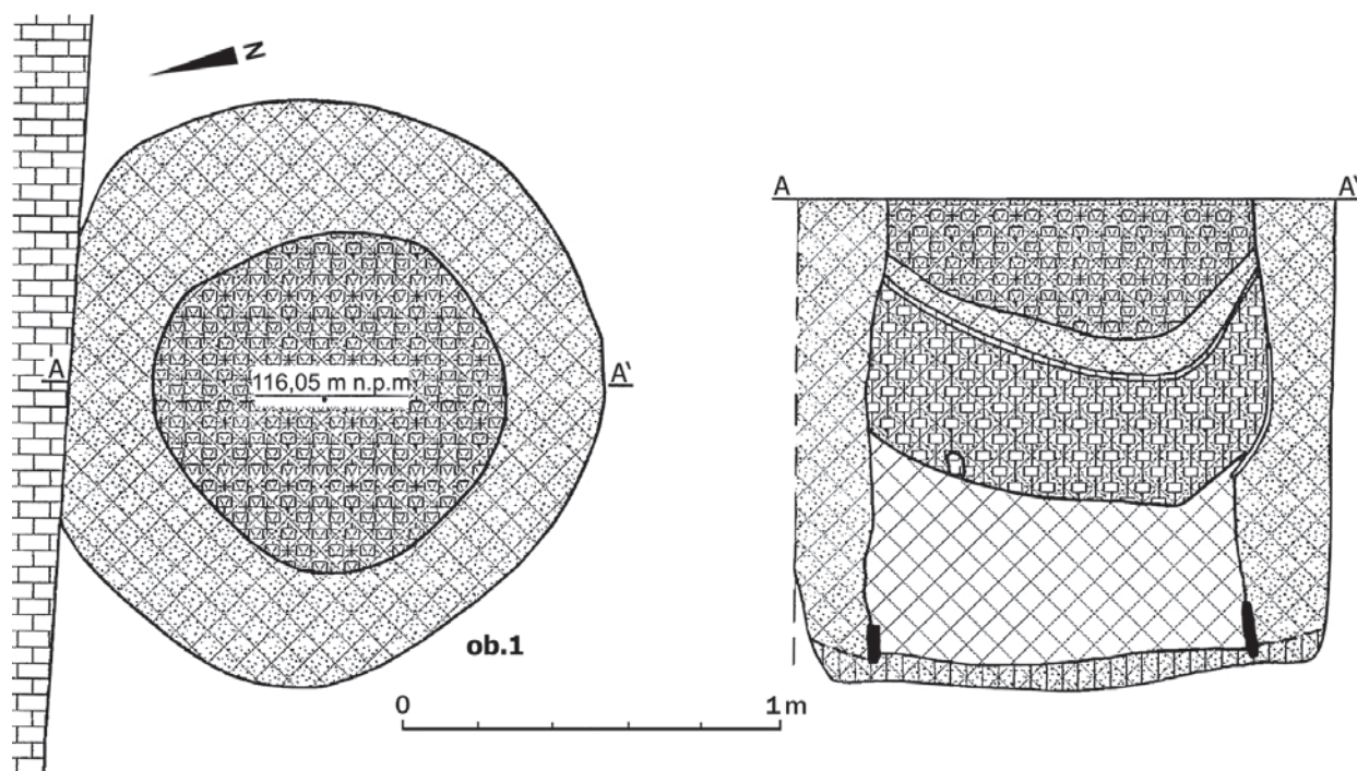
Ryc. 61. Ul. Wierzbowa 2, sektor 2, ob. 1 – jama garbarska. Rzut i profil. Wg M. Babija i in. (2001) Abb. 61. Weidenstraße 2, Sektor 2, Ob. 1 – Gerbergrube. Grundriss und Profil. Nach M. Babij et alii (2001)
