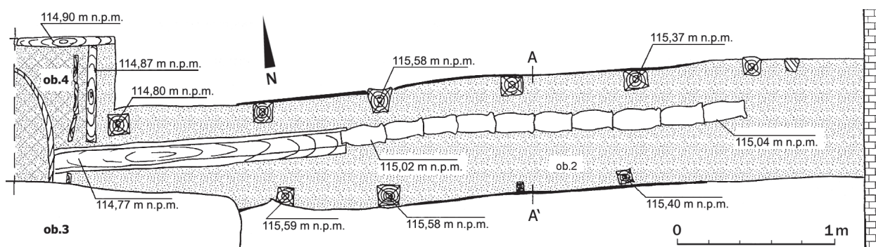
Ryc. 46. Ul. Biskupia 1a. Starszy wodociąg ceramiczny wraz z rzapiem (ob. 2 i 6).
