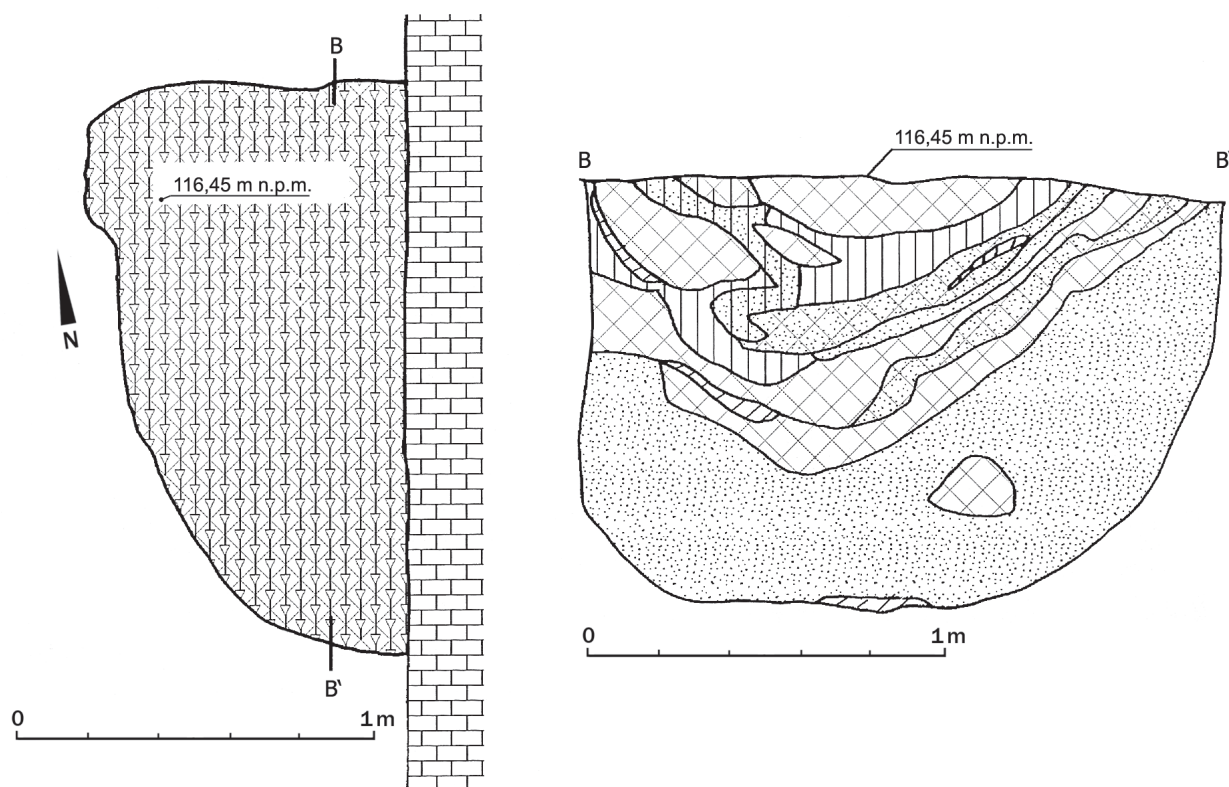
Ryc. 37. Ul. Oławska 69/ Biskupia 1-1a. Rzut i profil ziemianki (ob. 3). Rys. P. Konczewski Abb. 37. Altbüßerohle 69/ Bischofsgasse 1-1a. Grundriss und Profil der Grube (Ob. 3). Gezeichnet von P. Konczewski
