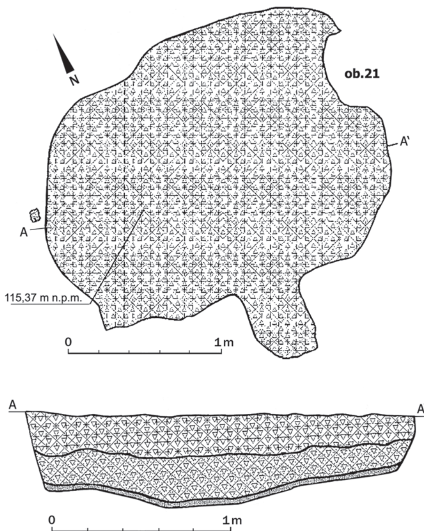
Ryc. 36. Ul. Ofiar Oświęcimskich 35. Rzut i profil piwniczki (ob. 21). Wg P. Guszpita i A. Limisiewicza (1998) Abb. 36. Junkernstraße 35. Grundriss und Profil des Kellers (Ob. 21). Nach P. Guszpit und A. Limisiewicz (1998)
