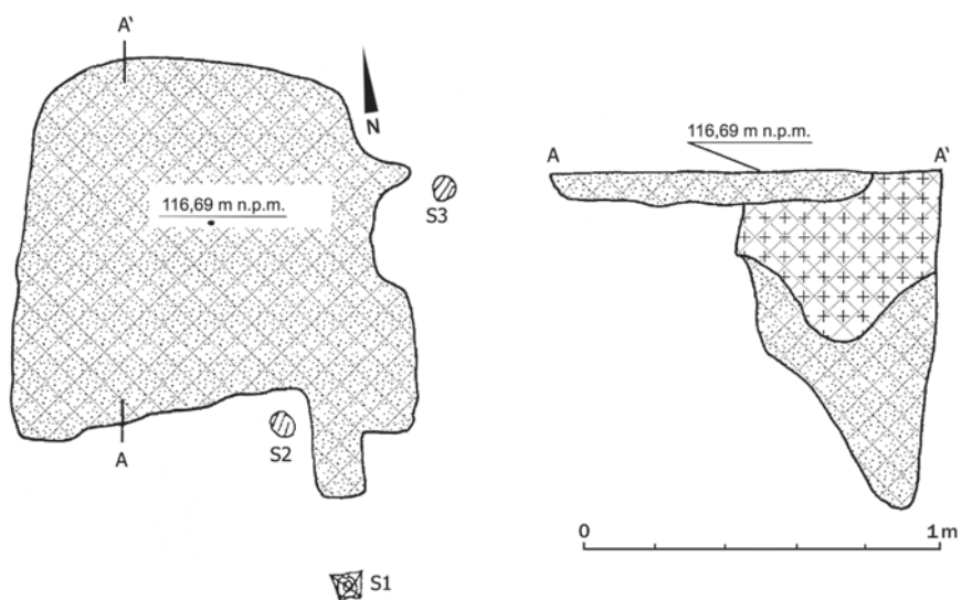
Ryc. 41. Ul. Biskupia 1a. Jama zasobowa ze śladami zadaszenia (ob. 4, sekt. 1). Rzut i profil. Wg M. Babija i in. (1999)
