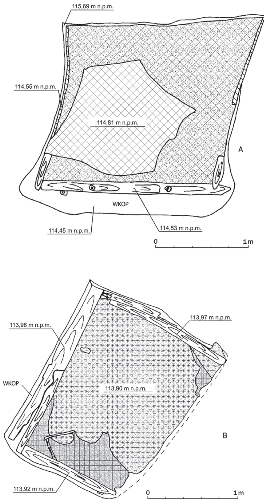
Ryc. 38. Ul. Kacerska Górka 13/ Nowa 36. Chłodnie odkryte na zapleczu parceli: A – ob. 1; B – ob. 2. Rys. P. Konczewski Abb. 38. Ketzberg 13/ Neue Gasse 36. Kühlräume auf dem Hinterhof: A – Ob. 1; B – Ob. 2. Gezeichnet von P. Konczewski
