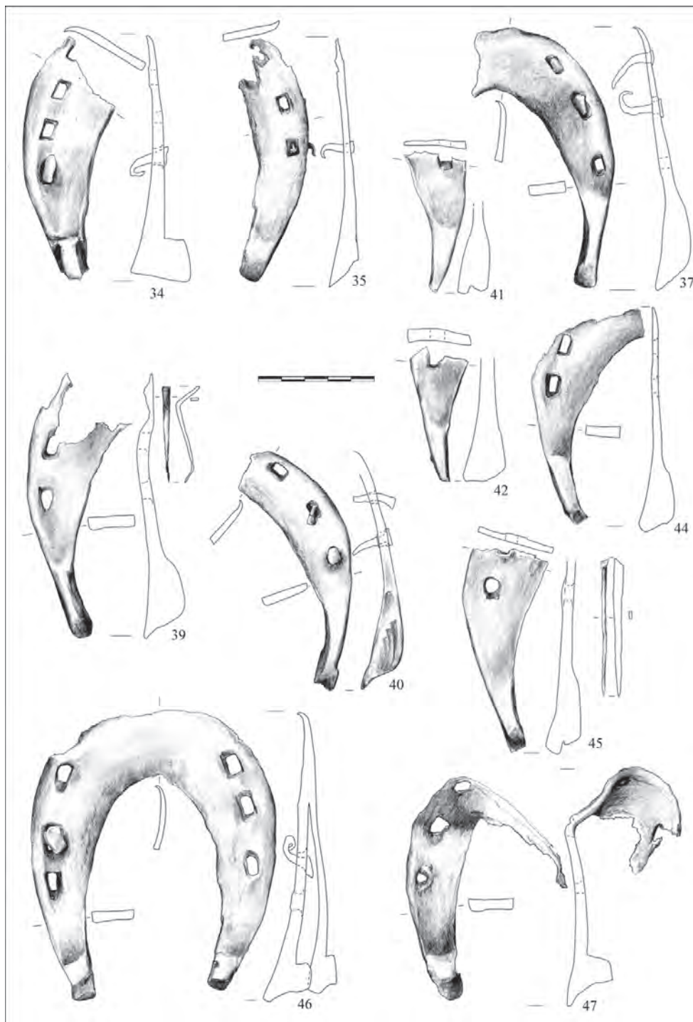
Ryc. 131. Wrocław, ul. Szewska. Podkowy żelazne: 34 – typ V/2; 35, 37, 39–42, 44–45 – typ VI/1; 46–47 – typ VI/2. Rys. N. Lenkow
