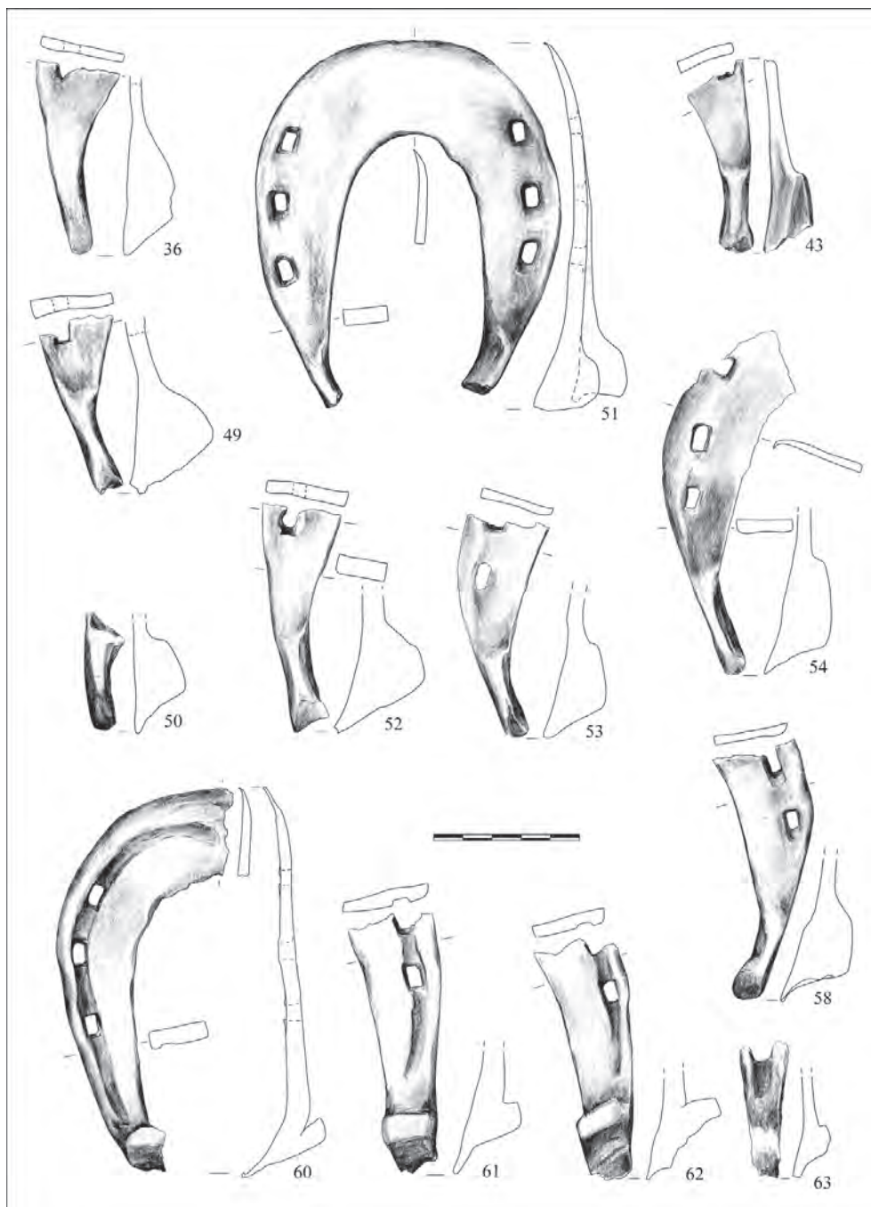
Ryc. 133. Wrocław, ul. Szewska. Podkowy żelazne: 36, 43 – typ VI/1; 49–54, 58 – typ VI/2; 60–63 – typ VI/4. Rys. N. Lenkow
