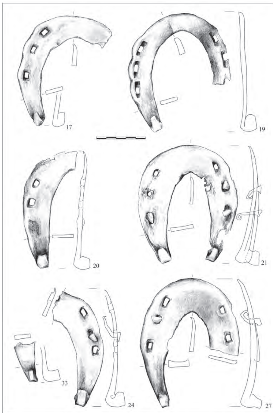
Ryc. 129. Wrocław, ul. Szewska. Podkowsy żelazne: 17 – typ III/2; 19 – typ III/4; 20 – typ IV/2; 21, 24, 27 – typ IV/3; 33 – nieokreślona odmiana typu IV. Rys. N. Lenkow
