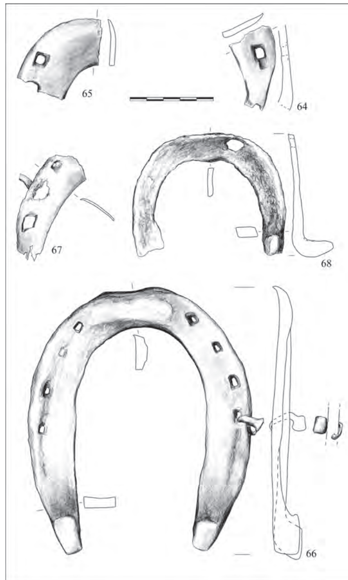
Ryc. 134. Wrocław, ul. Szewska. Podkowsy żelazne: 64 – nieokreślona odmiana typu VI; 65 – końska podkowska nieokreślonego typu IV–VII; 66 – końska podkowska nowożytna; 67 – podkowska osła lub muła (?); 68 – podkowska wołu (?). Rys. N. Lenkow
