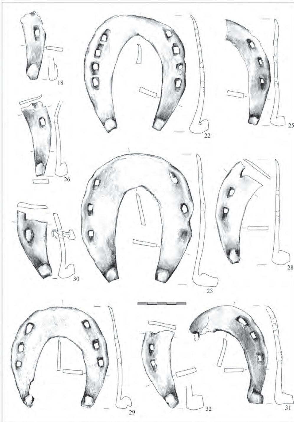
Ryc. 130. Wrocław, ul. Szewska. Podkowy żelazne: 18 – typ III/2; 22–23, 25–26, 28–32 – typ IV/3. Rys. N. Lenkow Fig. 130. Wrocław, Szewska St. Iron horseshoes: 18 – type III/2; 22–23, 25–26, 28–32 – type IV/3. Drawing N. Lenkow
