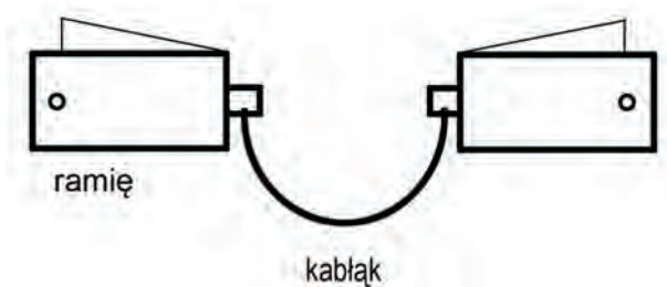
Ryc. 6. Konstrukcja okucia kabłąkowego, rys. Jakub Sawicki
