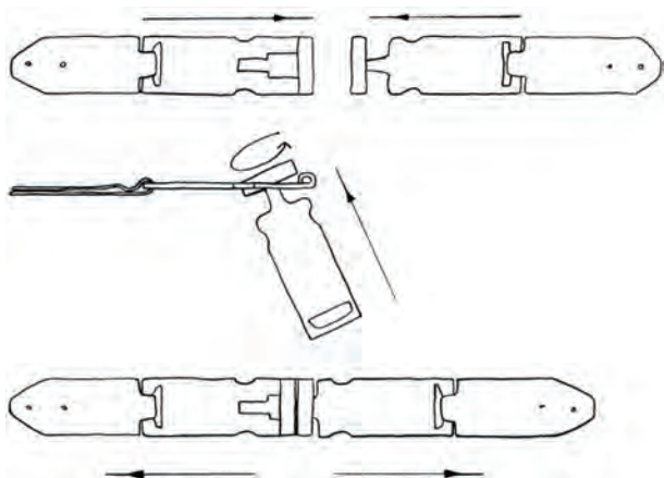
Ryc. 4. Konstrukcja i sposób działania zapięcie szczelinowego, za: Harder 2010, s. 6, ryc. 10
