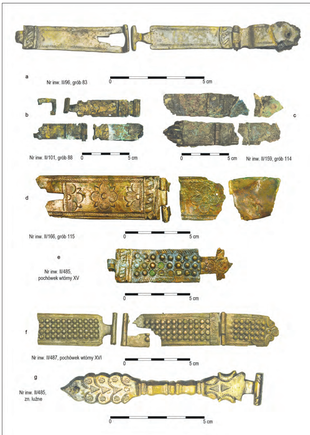
Tabl. 5. Wrocław, cmentarz Salwatora. Zapięcia szczelinowe. Fot. J. Wojcieszak Table 5. Wrocław, cemetery of Our Saviour. Slot buckles. Photo by J. Wojcieszak
